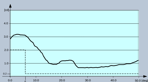
Fig. 1 OACI par. 5.3.18.8 e FAA L-852T – Blu
