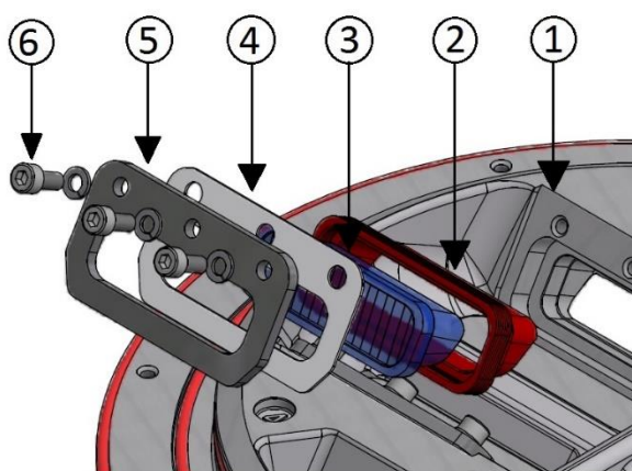
Figura 24 – Guarnizioni del prisma
