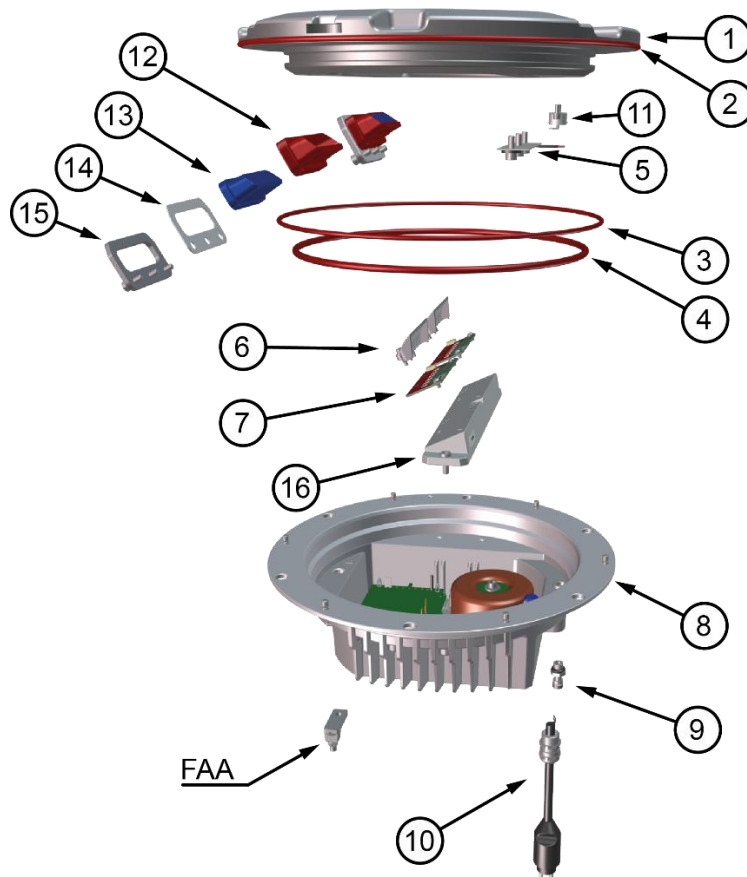
Figura 5 – Vista esplosa
