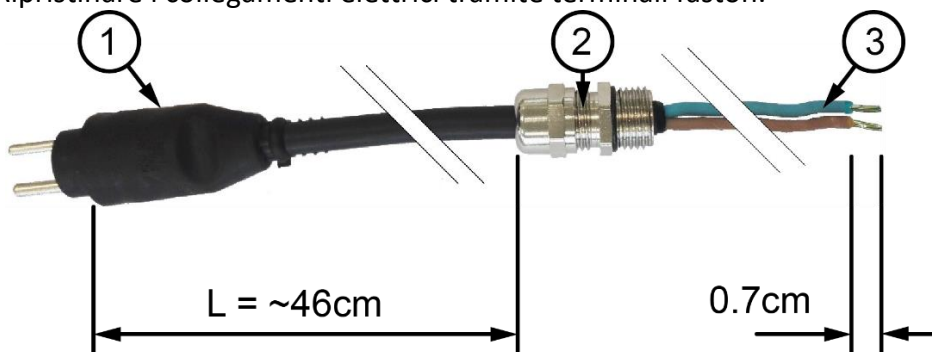
Figura 25 – Cavetto di Alimentazione con Spina
