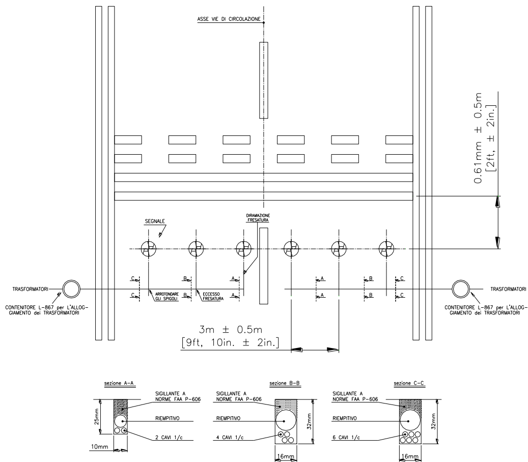
Figura 10 – Esempio di Disposizione dei Segnali
