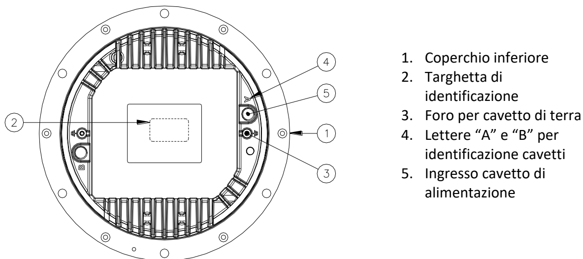
Figura 2 – Coperchio inferiore - vista esterna
