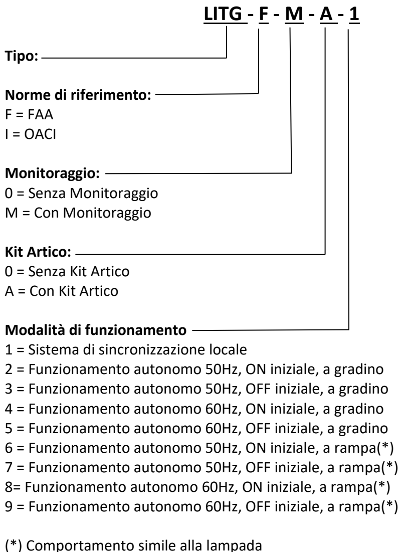
Figura 7 - Identificazione del P/N completo
