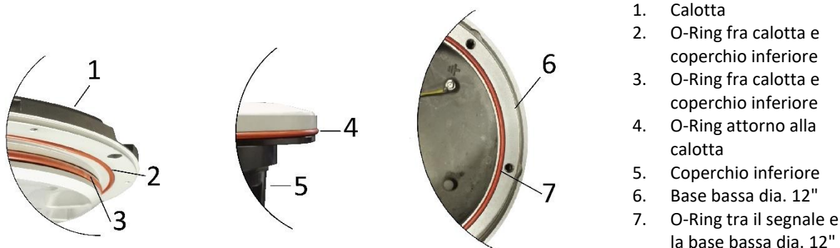
Figura 23– Guarnizioni del segnale
