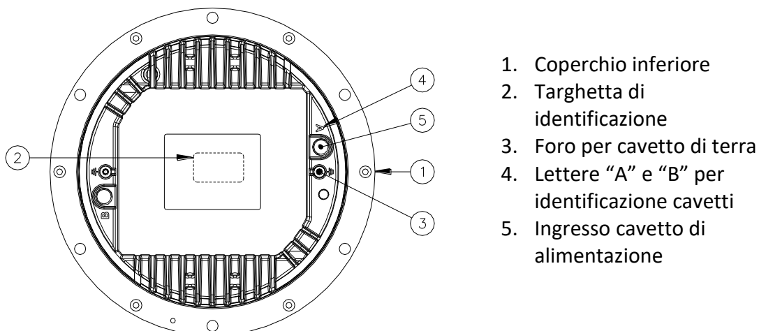
Figura 2 – Coperchio inferiore - vista esterna
