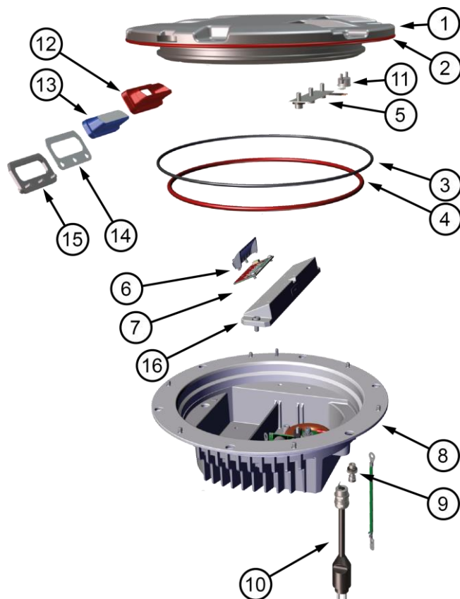
Figura 5 – Vista esplosa
