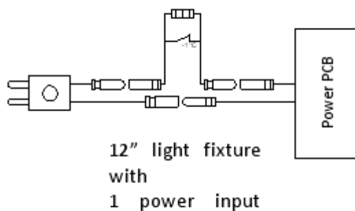
Figura 23 – Schema di collegamento elettrico del kit artico
