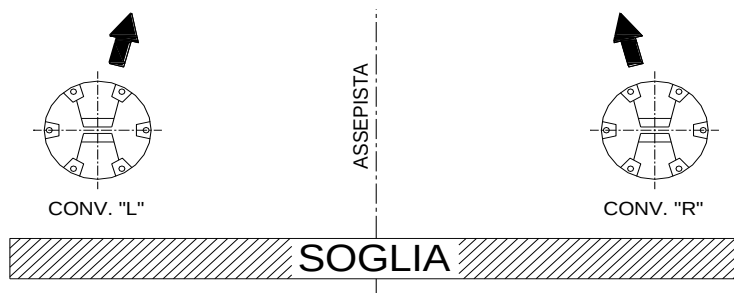
Figura 7 - Identificazione del P/N completo
