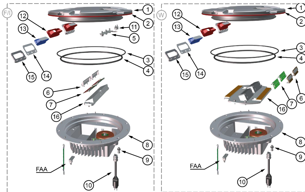
Figura 5 – Vista esplosa, LIRT soglia (sx), LIRT ali di soglia (dx)
