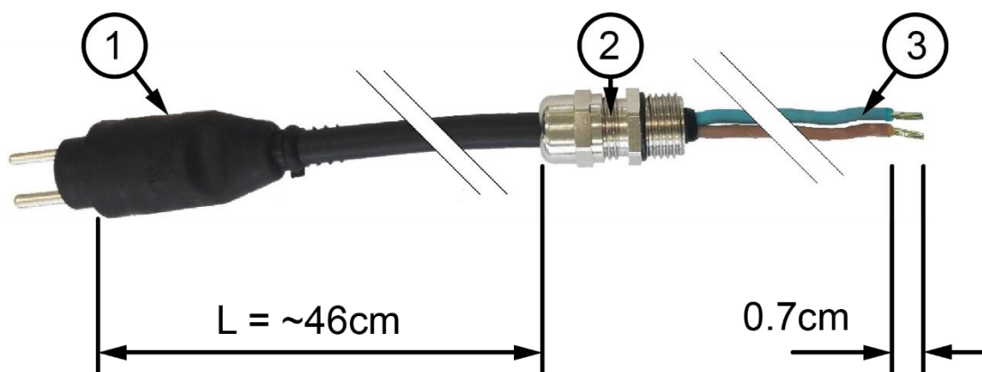
Figura 26 – Cavetto di Alimentazione con Spina
