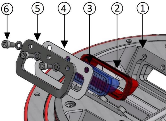
Figura 25 – Guarnizioni del prisma
