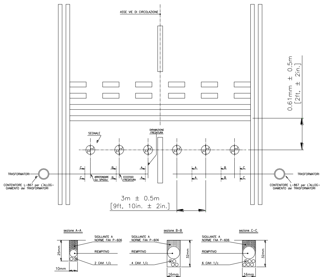
Figura 10 – Esempio di Disposizione dei Segnali
