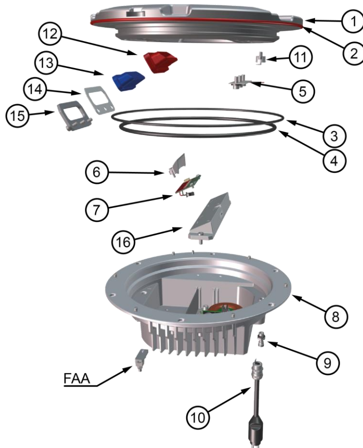
Figura 5 – Vista esplosa
