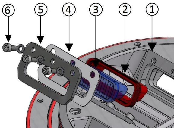
Figura 20 – Sostituzione del prisma
