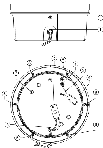
Figura 8 – Base Basso Standard 12"
