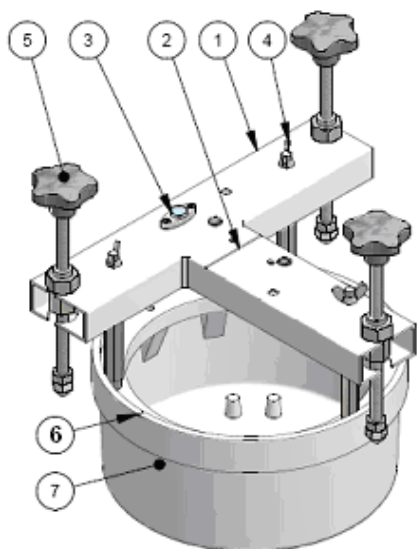
Figura 12 – Base da 12" per canalizzazione laterale o dal fondo (metodo B)
