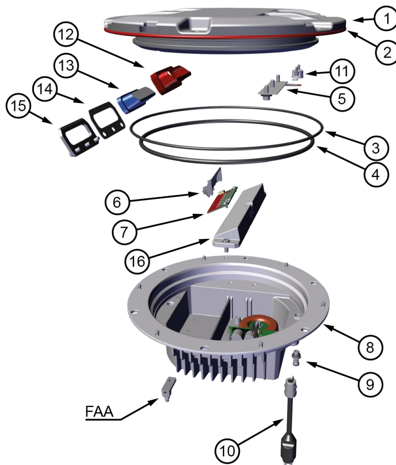
Figura 5 – Vista esplosa
