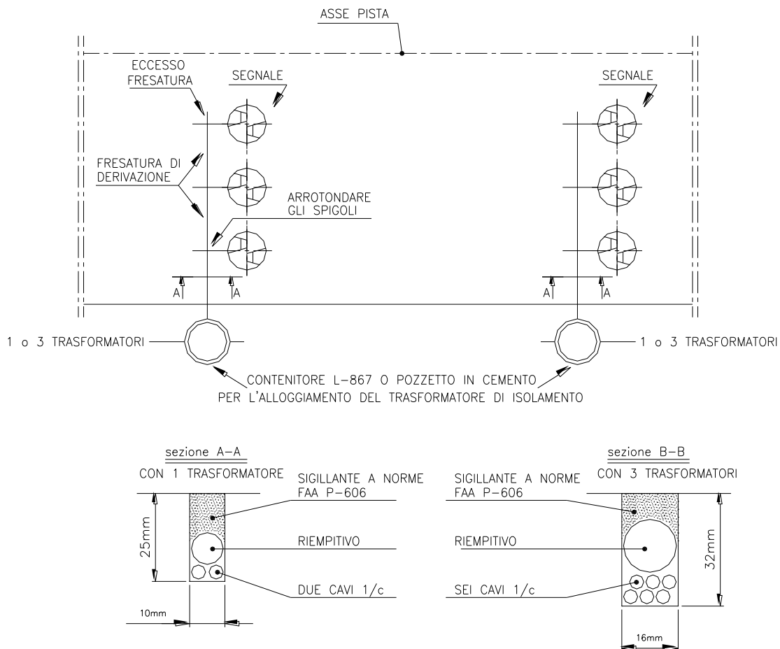
Figura 10 – Esempio di Disposizione dei Segnali
