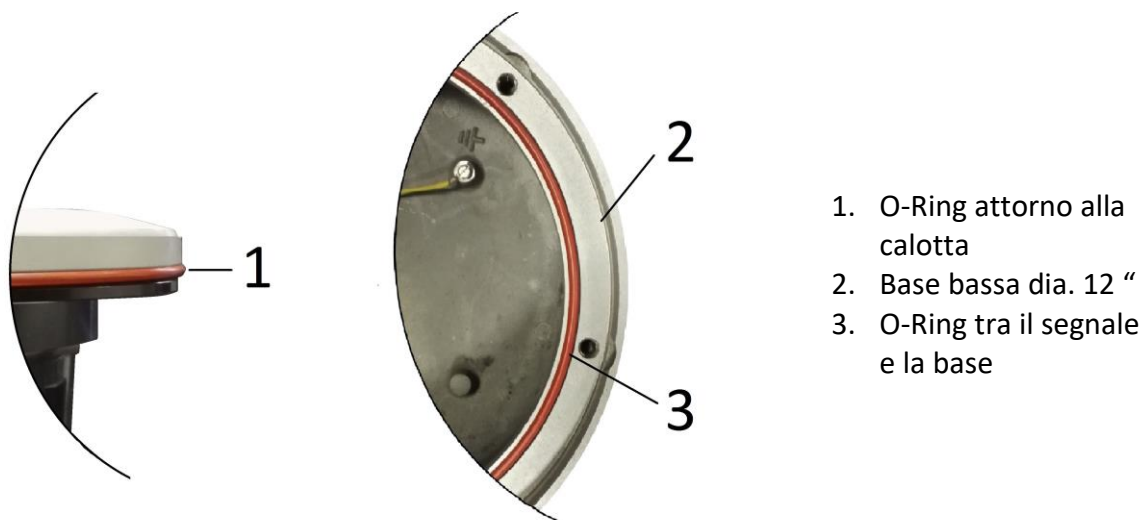
Figura 12 – Guarnizione per base bassa standard 12''
