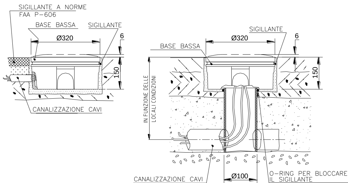
Figura 13 – Base da 12'' per canalizzazione laterale o dal fondo (metodo B)
