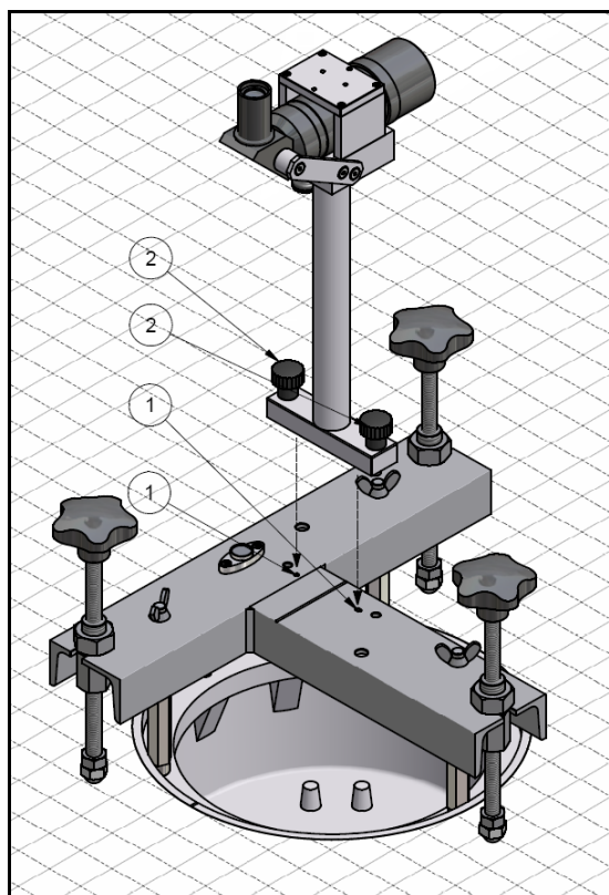
Figura 15 – Dispositivo ottico (fare riferimento al manuale UT-MT-0485 per ulteriori informazioni)
