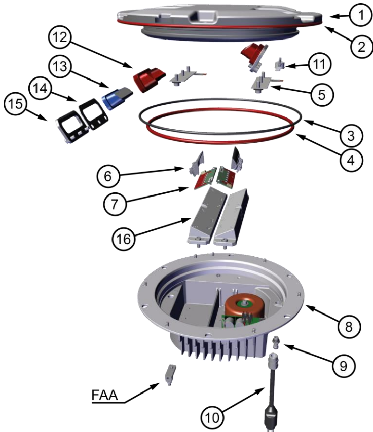
Figura 5 – Vista esplosa
