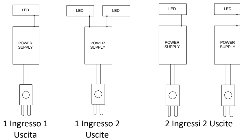
Figura 4 – Schema Elettrico
