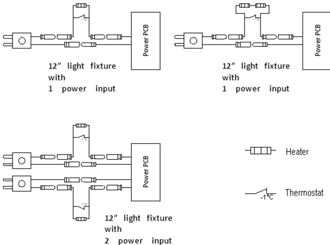
Figura 23 – Schema di collegamento elettrico del kit artico
