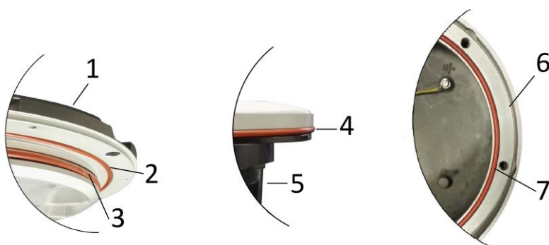
Figura 19 – Guarnizioni del segnale
