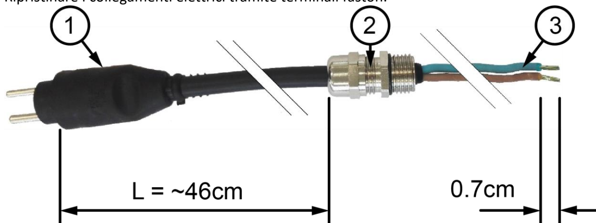
Figura 26 – Cavetto di Alimentazione con Spina
