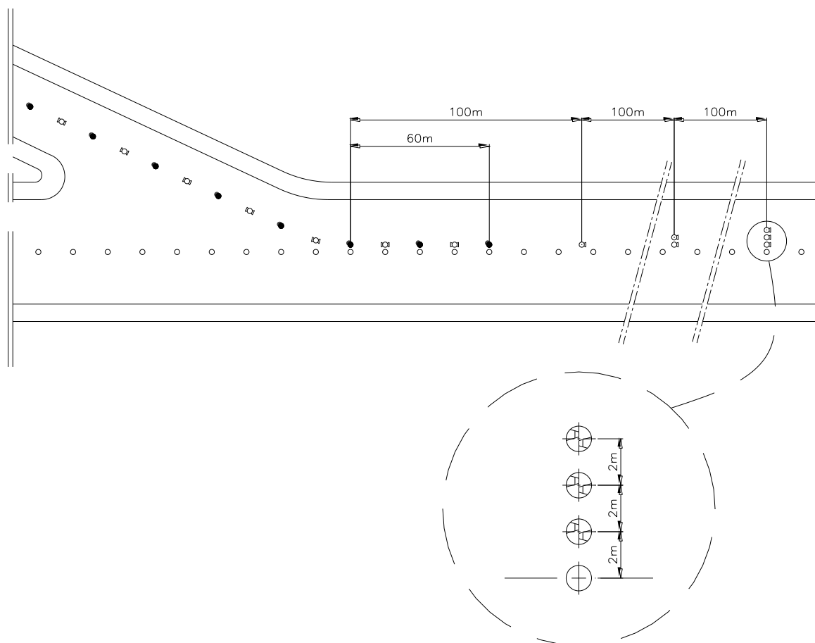
Figura 11 – Disposizione per segnali R.E.T.I.L.
