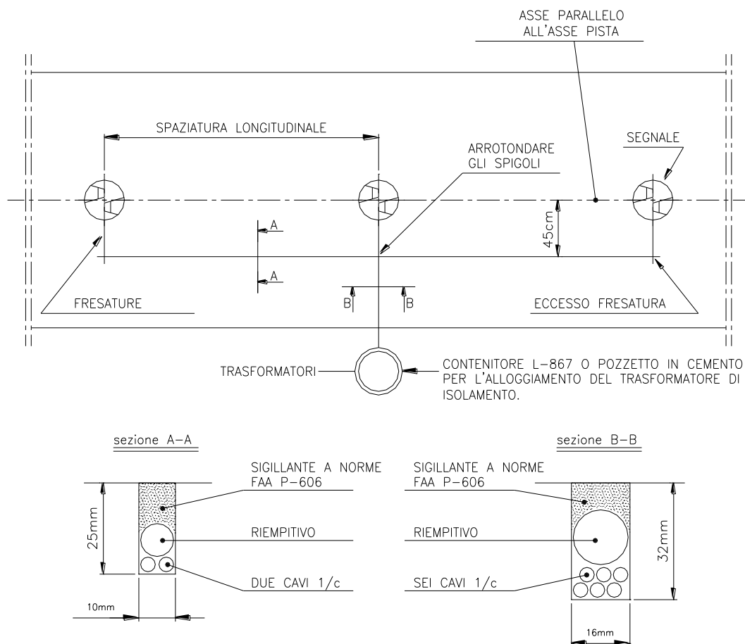
Figura 10 – Esempio di Disposizione dei Segnali (Un Trasformatore per ogni Segnale)
