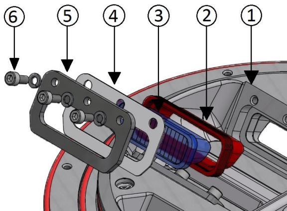
Figura 21 – Sostituzione del prisma
