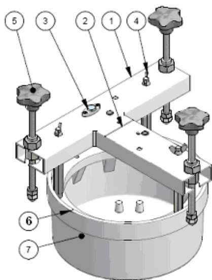
Figura 14 – Dettagli di installazione della base bassa
