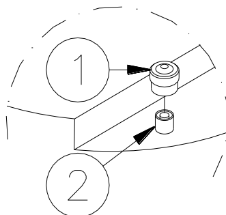
Figura 21 – Coperchio inferiore con valvola di pressione
