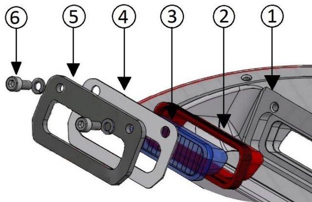
Figura 24 – Sostituzione del prisma
