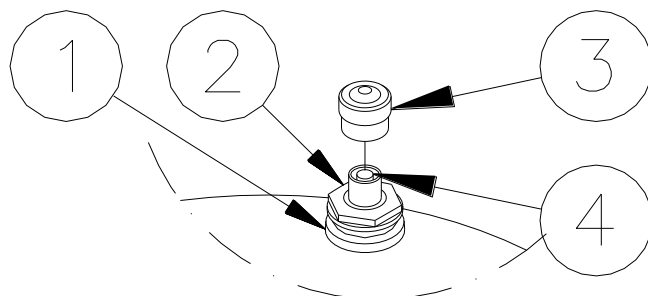
Figura 30 – Copertura inferiore con valvola di pressione
