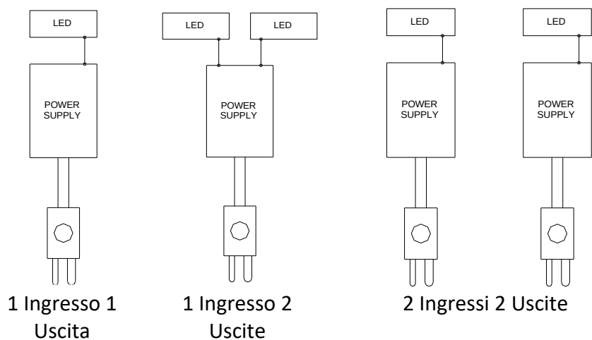
Figura 4 – Schema Elettrico
