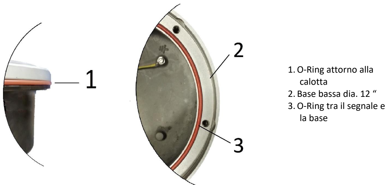
Figura 14 – Guarnizione per base bassa standard 12"
