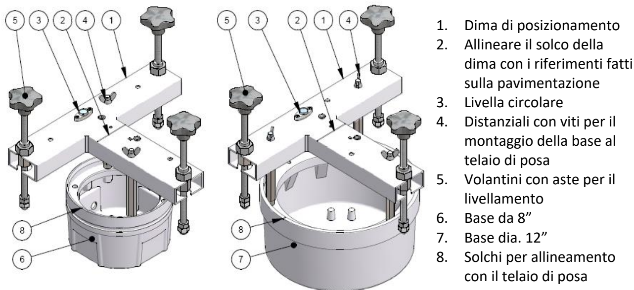
Figura 17 – Dettagli di installazione della base bassa
