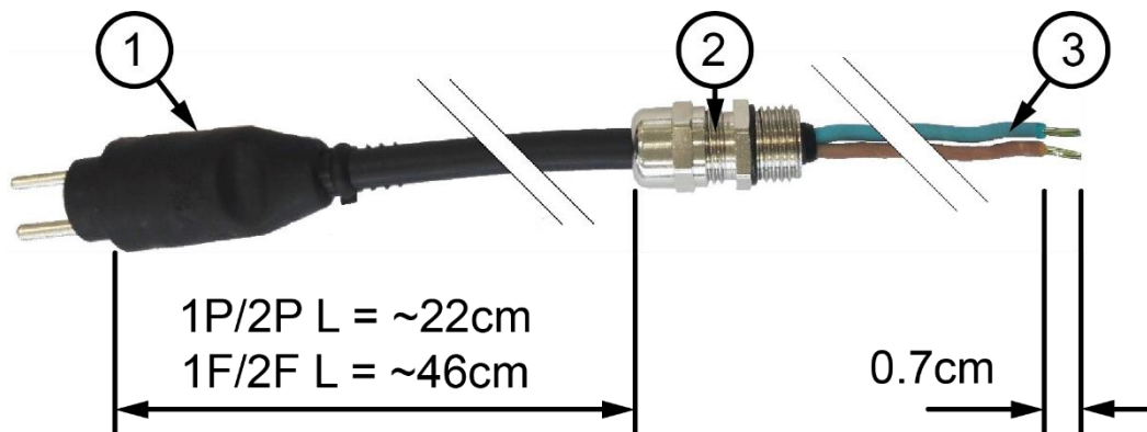
Figura 29 - Cavetto di alimentazione unipolare con spina
