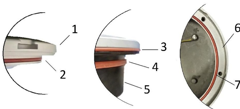
Figura 22 – Guarnizioni del segnale
