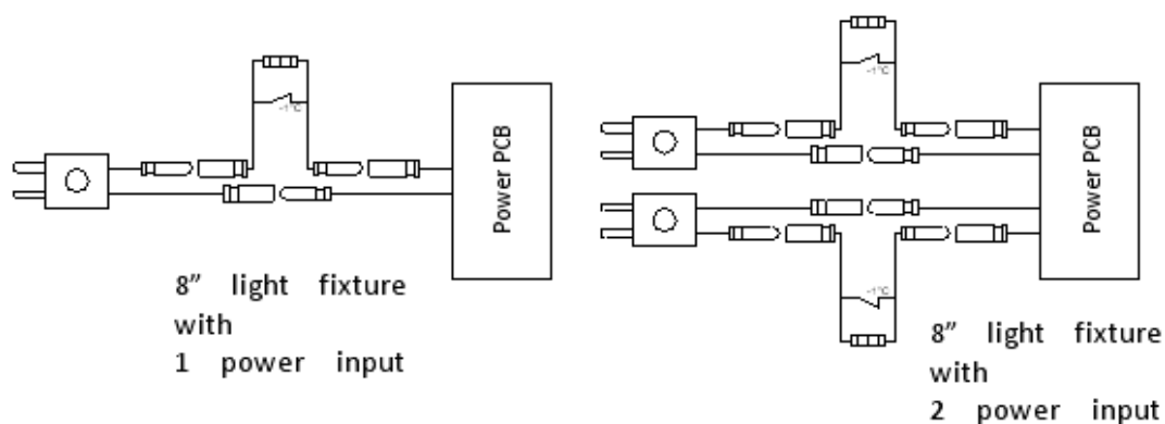
Figura 26 – Schema di collegamento elettrico del kit artico
