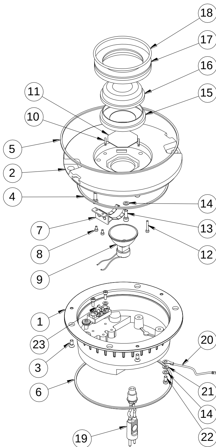
Figura 5 – Vista esplosa
