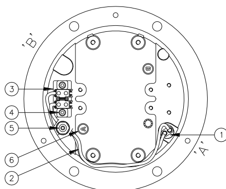
Figura 3 – Coperchio inferiore - vista interna
