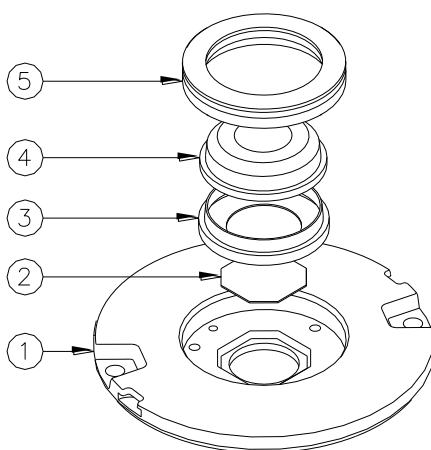
Figura 28 – Guarnizione del prisma
