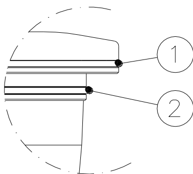
Figura 11 – Guarnizione per base bassa standard 8"
