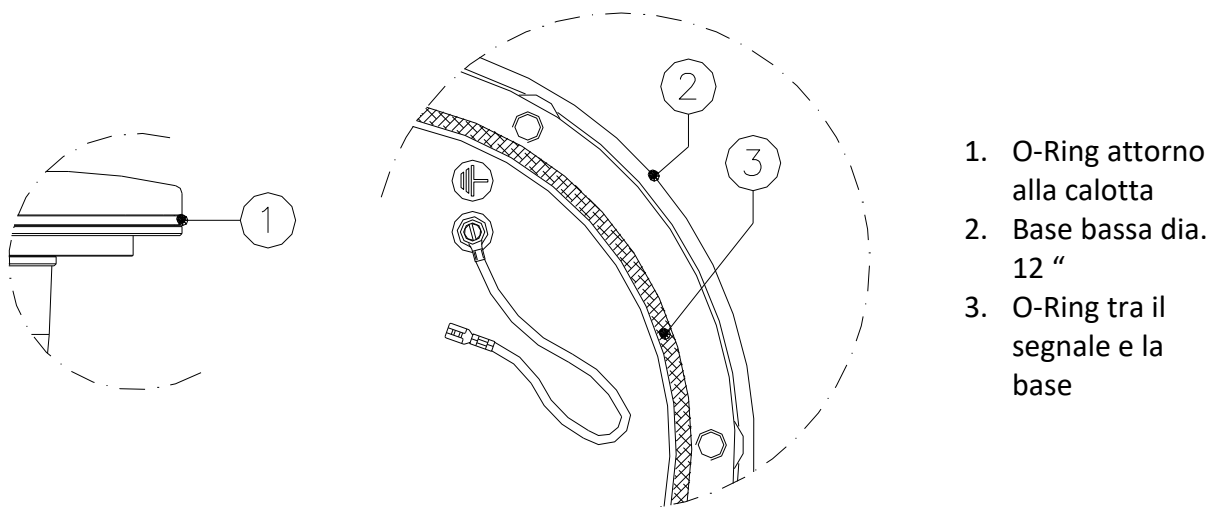
Figura 12 – Guarnizione per base bassa standard 12"
