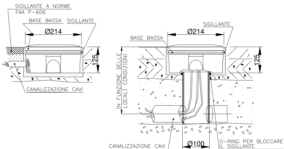
Figura 16 – Base da 8" per canalizzazione laterale o dal fondo (metodo B)
