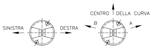
Orientamento per tratti dritti e tratti curvi
