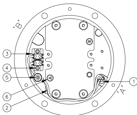
Figura 3 – Coperchio inferiore - vista interna
