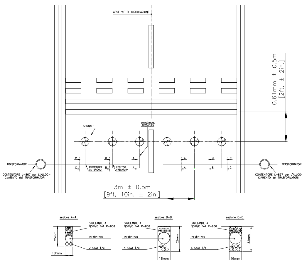
Figura 12 – Barre d'Arresto (OACI) Schema di Disposizione dei Segnali
