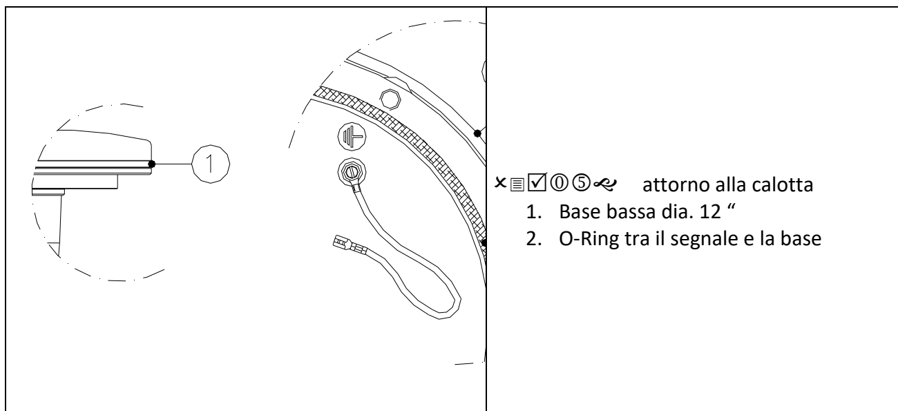
Figura 15 – Guarnizione per base bassa standard 12"
