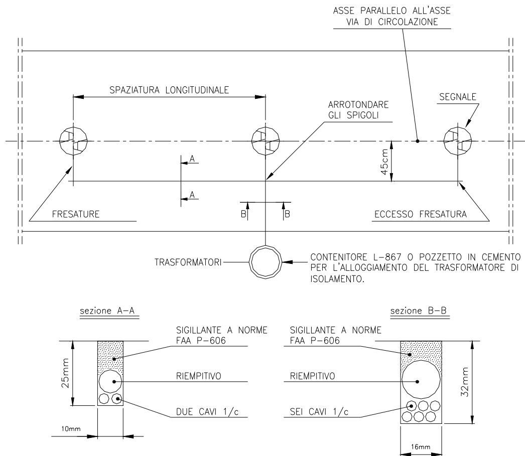
Figura 11 – Asse Vie di Circolazione (OACI) Schema di Disposizione dei Segnali
