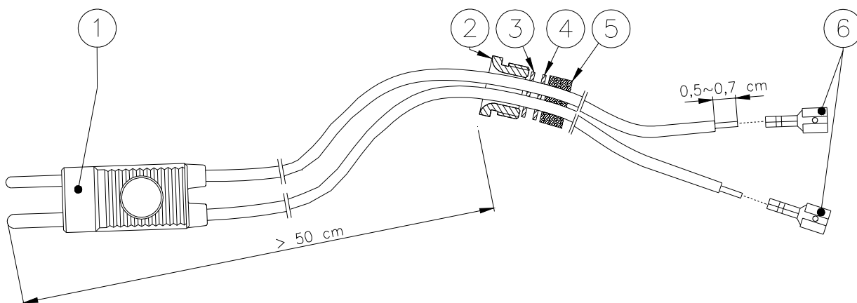
Figura 33 – Cavetto di Alimentazione con Spina
