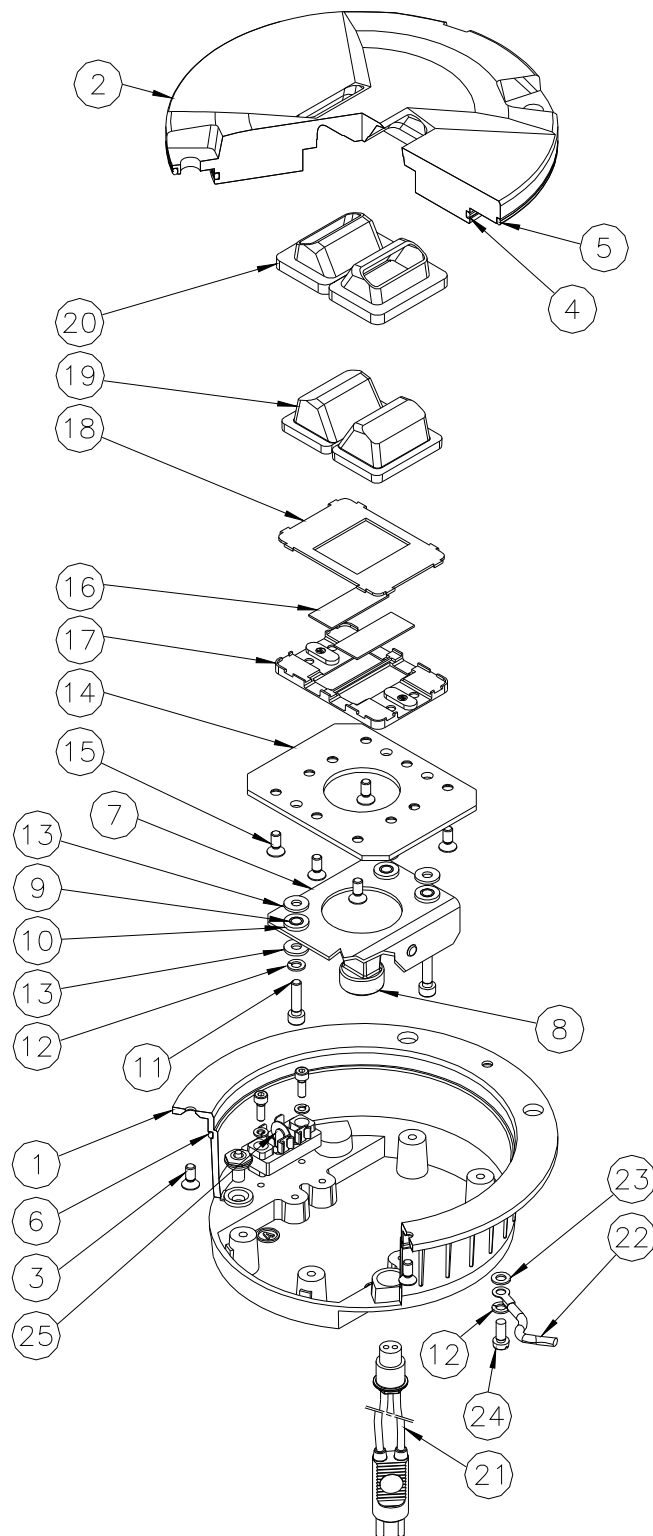
Figura 5 – Vista esplosa
