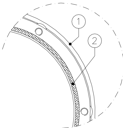
Figura 20 – Guarnizione per base L-868
