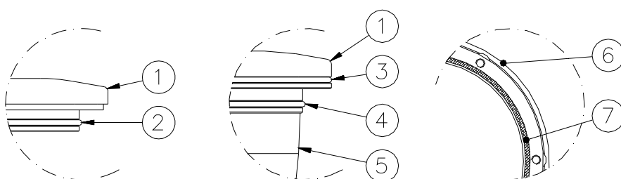
Figura 30– Guarnizioni del segnale
