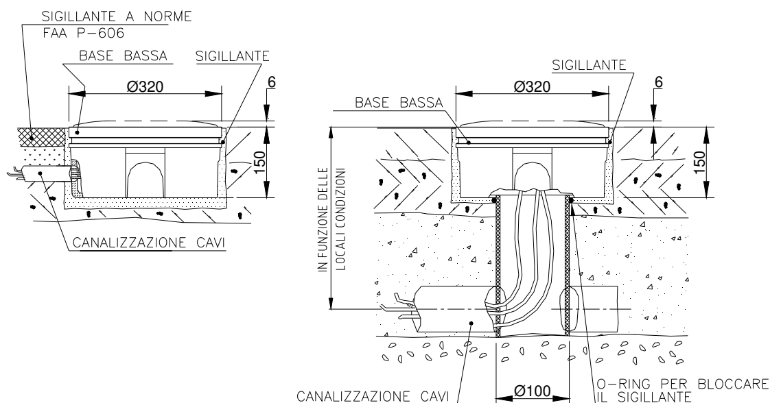
Figura 17 – Base da 12" per canalizzazione laterale o dal fondo (metodo B)
