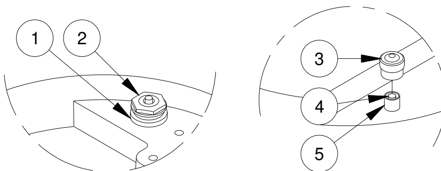
Figura 34 – Copertura inferiore con valvola di pressione
