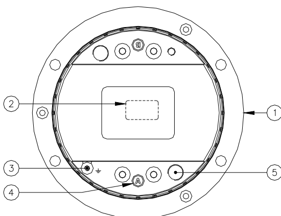
Figura 2 – Coperchio inferiore - vista esterna
