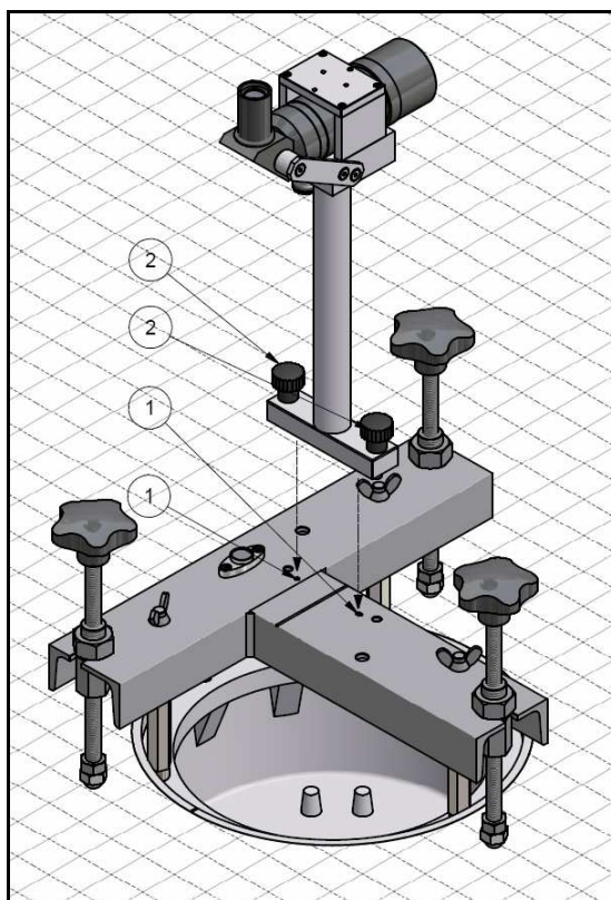
Figura 19 – Dispositivo ottico (fare riferimento al manuale UT-MT-0485 per ulteriori informazioni)
