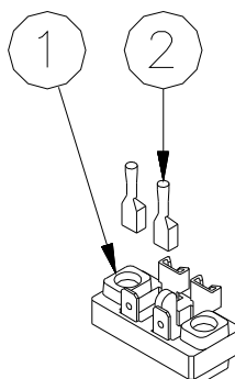
Figura 32 – Faston Femmina della Basetta Isolante
