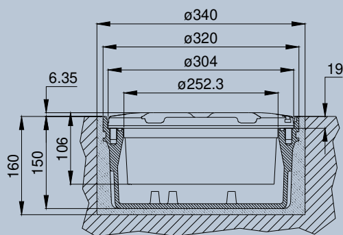
Base peu profonde de 12" de diamètre
