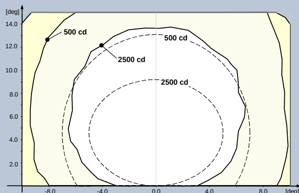
Рис. 3 FAA L-850A – Белый
