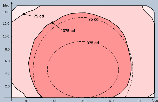
Рис. 4 FAA L-850A – Красный
