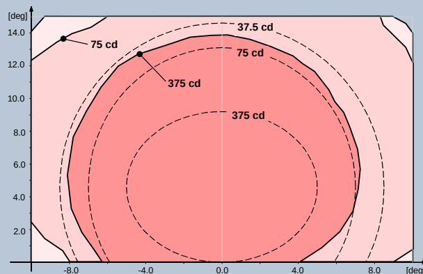
Рис. 2 ICAO A2-7 15 м – Красный
