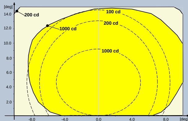
Рис. 6 ICAO A2-7 R.E.T.I.L. – Желтый
