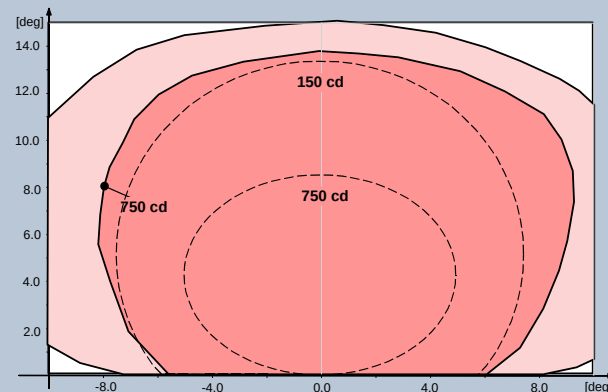
Рис. 5 FAA L-850T – Красный
