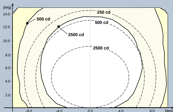
Рис. 1 ICAO A2-7 15 м – Белый
