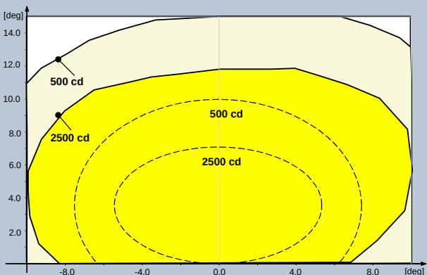
Fig. 5 FAA L-850C – Amarillo
