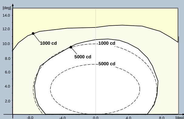
Fig. 3 FAA L-850C – Blanco
