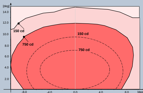
Fig. 4 FAA L-850C – Rojo
