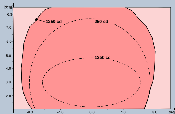
Fig. 4 FAA L-850D – Rosso
