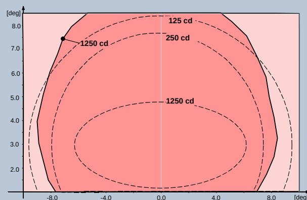
Fig. 2 OACI A2-8 – Rosso
