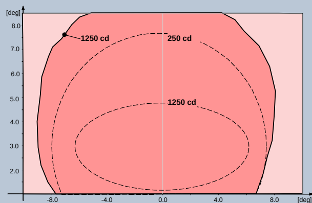
Abb. 4 FAA L-850D – Rot
