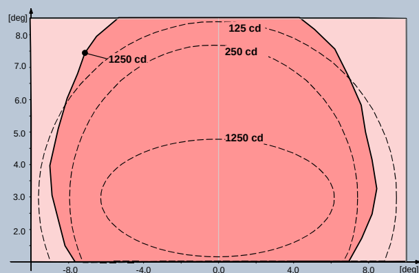
Abb. 2 OACI A2-8 – Rot
