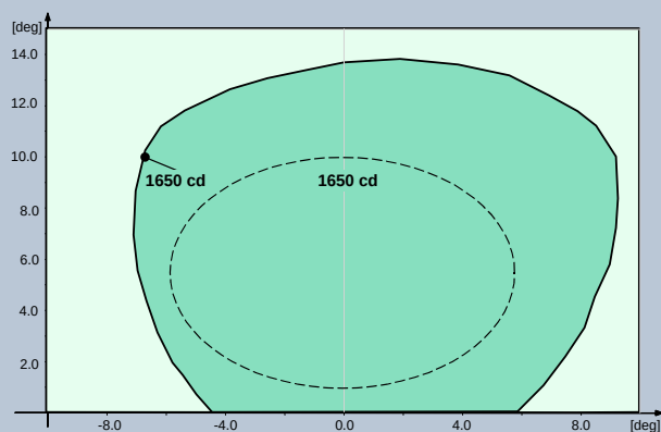
Abb. 3 FAA L-850D – Grün
