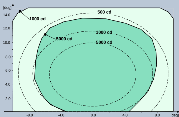
Abb. 1 OACI A2-3 – Grün
