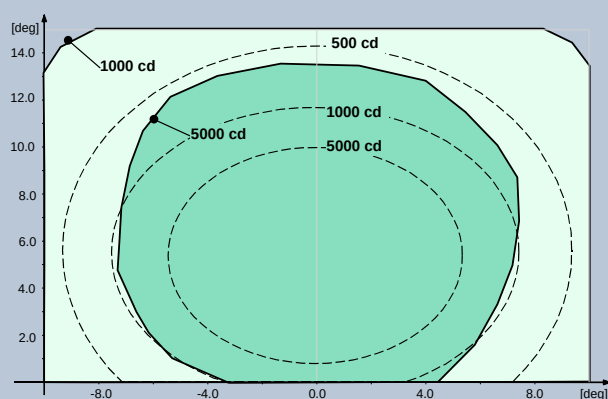
Fig. 1 Soglia OACI A2-3 – Verde
