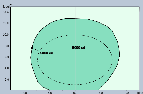
Fig. 2 Soglia FAA L-850E – Verde
