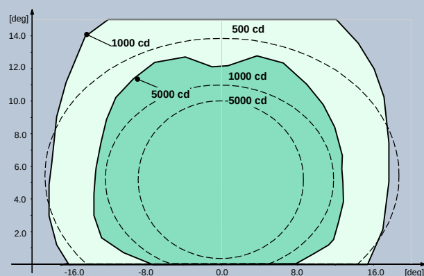
Fig. 3 Ali di Soglia OACI A2-4 – Verde
