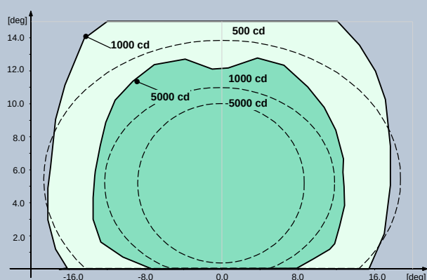
Fig. 3 Barres de Flanc de Seuil ICAO A2-4 – Vert
