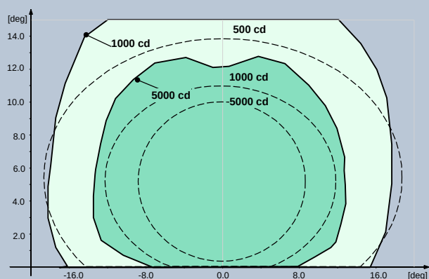
Fig. 3 Barra de Ala de Umbral OACI A2-4 – Verde
