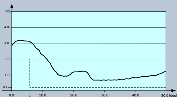
Fig. 1 OACI par. 5.3.17.8 e FAA L-852T – Blu
