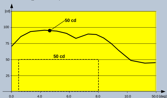
Fig. 2 FAA L-852E – Giallo
