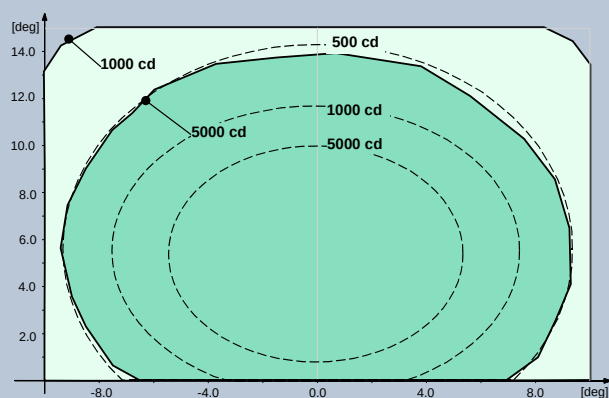
Fig. 1 OACI A2-3 – Vert
