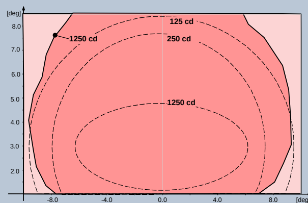
Fig. 2 OACI A2-8 – Rouge
