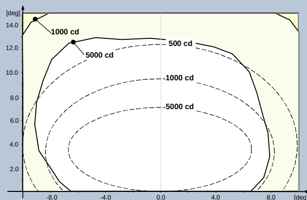
Fig. 2 OACI A2-10 60 m – Blanc
