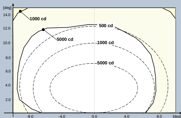
Fig. 1 OACI A2-9 45 m – Blanc
