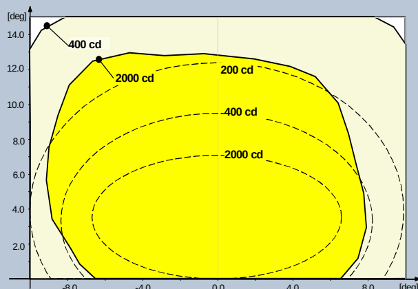
Fig. 3 OACI A2-10 60 m – Jaune
