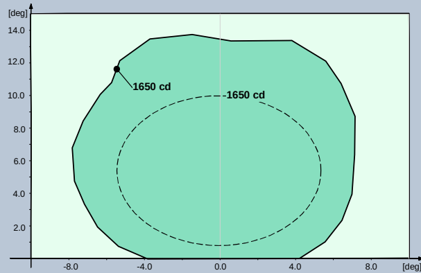
Fig. 6 FAA L-850D – Vert
