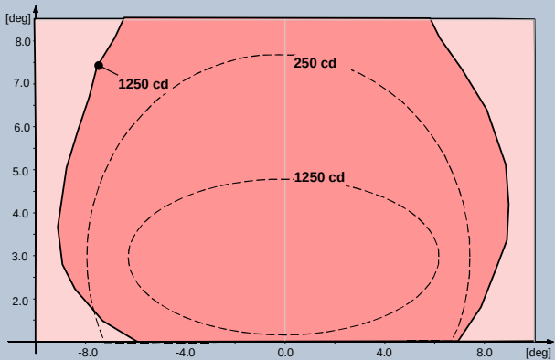
Fig. 7 FAA L-850D – Rouge
