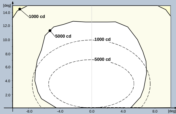
Fig. 5 FAA L-850C – Blanc
