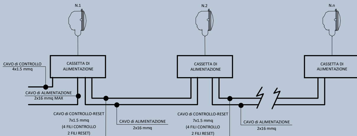
SISTEMA LAMPEGGIANTE A TRE LIVELLI
