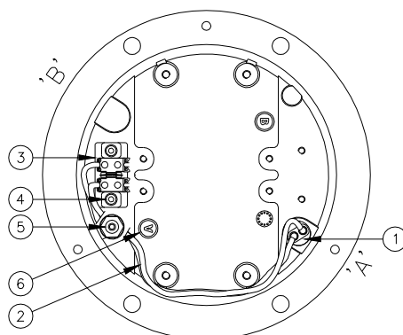
Figura 3 – Coperchio inferiore - vista interna
