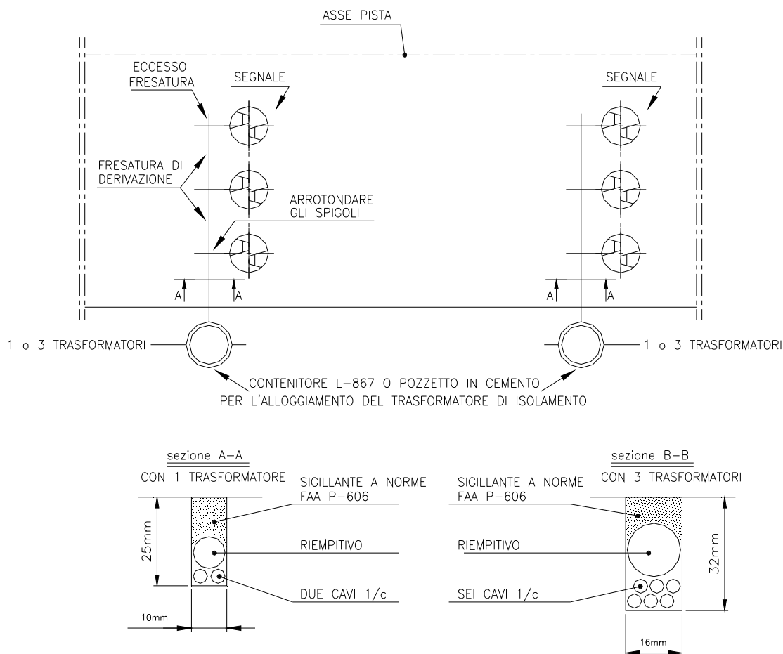
Figura 11 – Esempio di Disposizione dei Segnali
