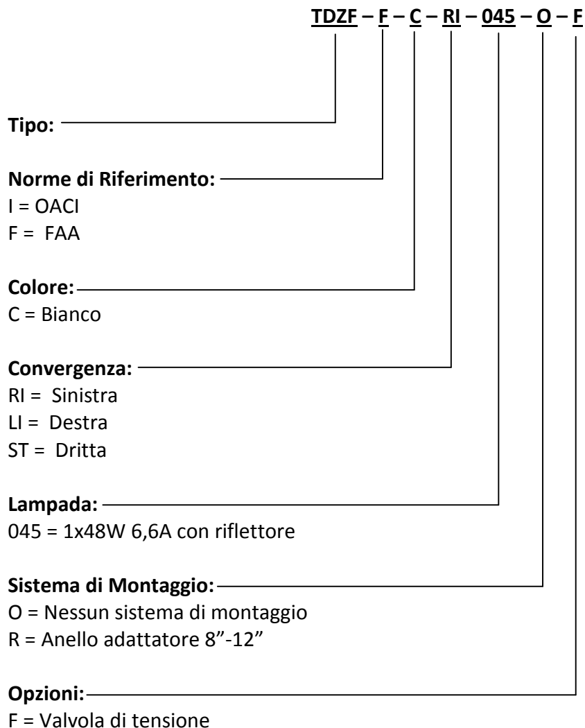
Figura 7 – Identificazione del P/N completo
