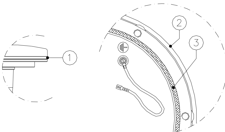
Figura 12 – Guarnizione per base bassa standard 8”
