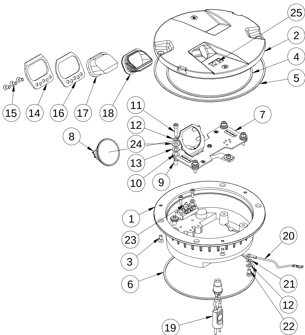
Figura 5 – Vista esplosa
