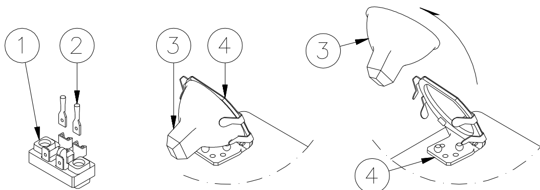
Figura 25 – Sostituzione lampada
