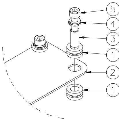
Figura 30 – Supporto Antivibrante
