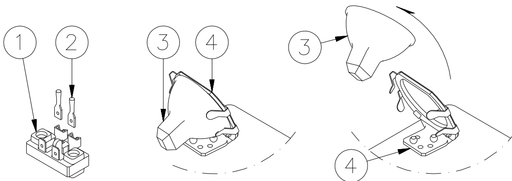
Figura 25 – Sostituzione lampada
