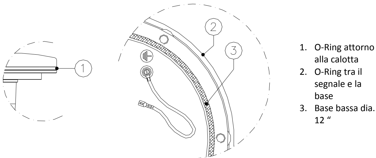
Figura 13 – Guarnizione per base bassa standard 12"
