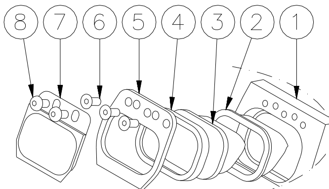
Figura 23 – Sostituzione del prisma
