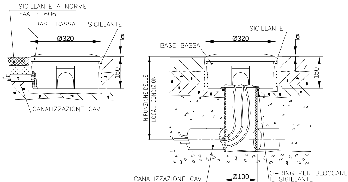
Figura 15 – Base da 12" per canalizzazione laterale o dal fondo (metodo B)
