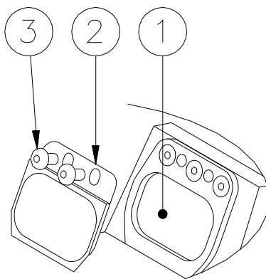
Figura 22 – Pulizia del prisma
