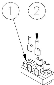
Figura 28 – Faston Femmina della Basetta Isolante
