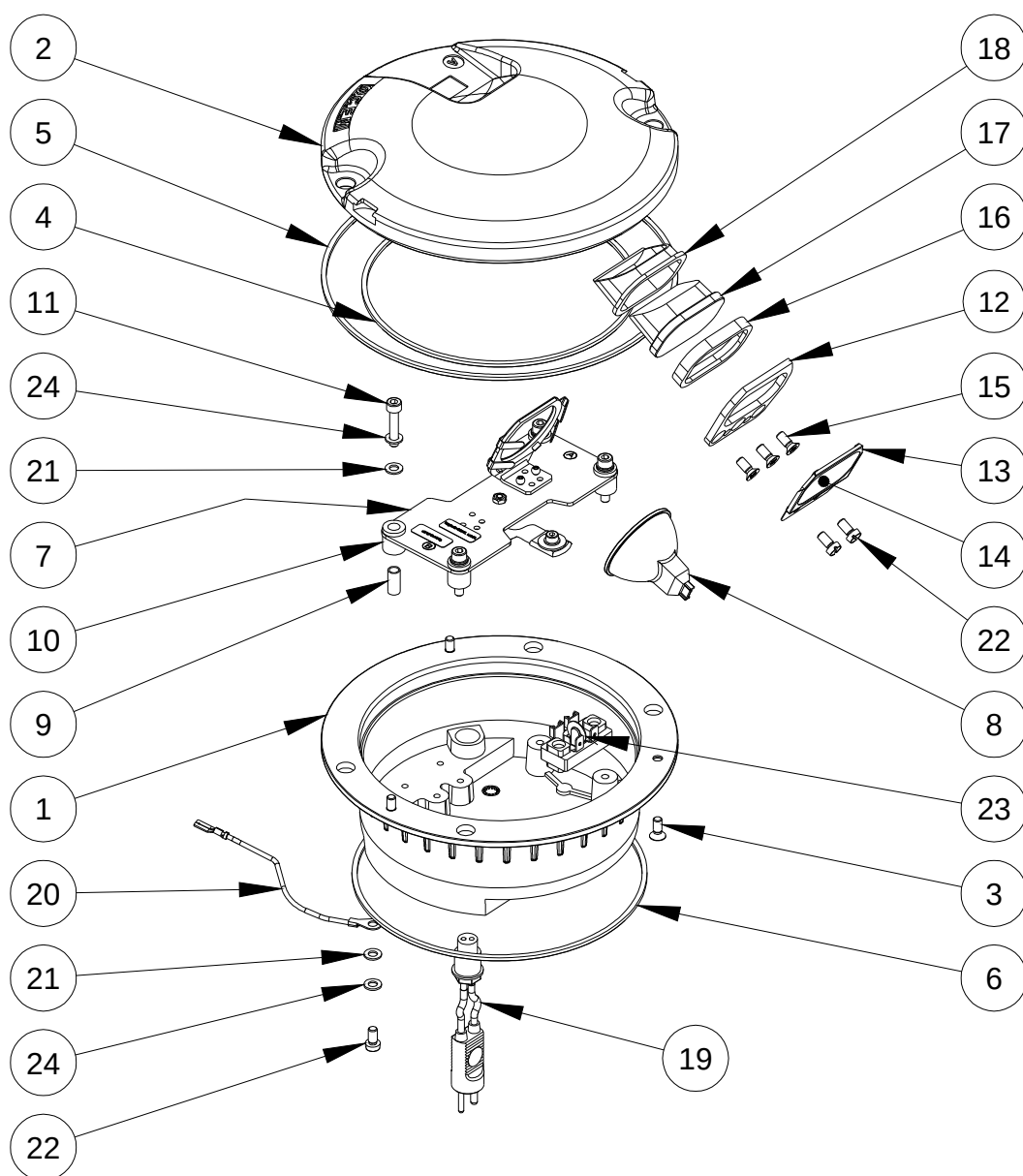
Figura 5 – Vista esplosa
