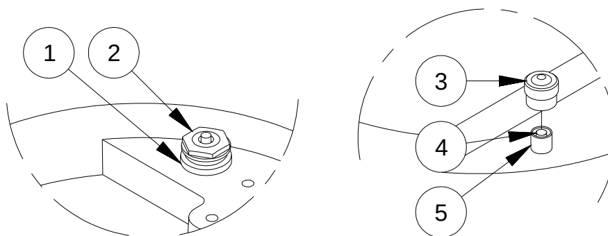
Figura 31 – Copertura inferiore con valvola di pressione
