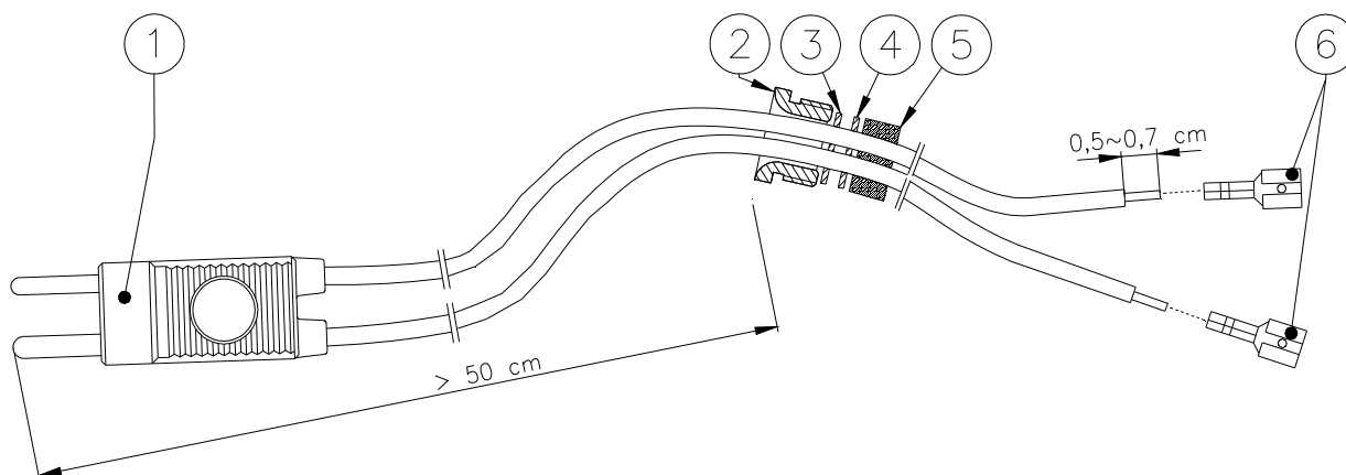
Figura 29 – Cavetto di Alimentazione con Spina
