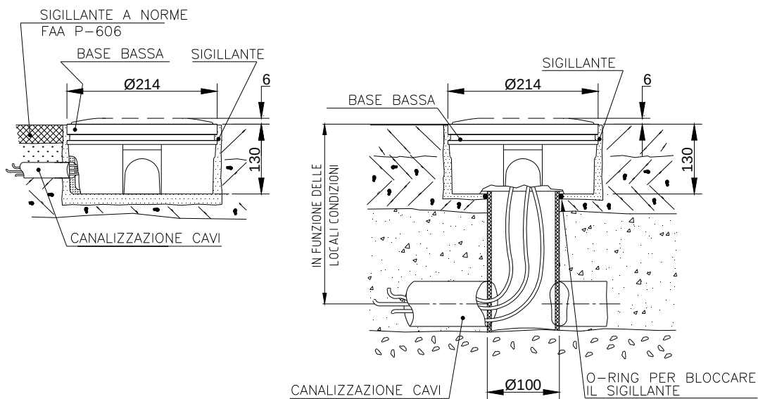
Figura 14 – Base da 8" per canalizzazione laterale o dal fondo (metodo B)
