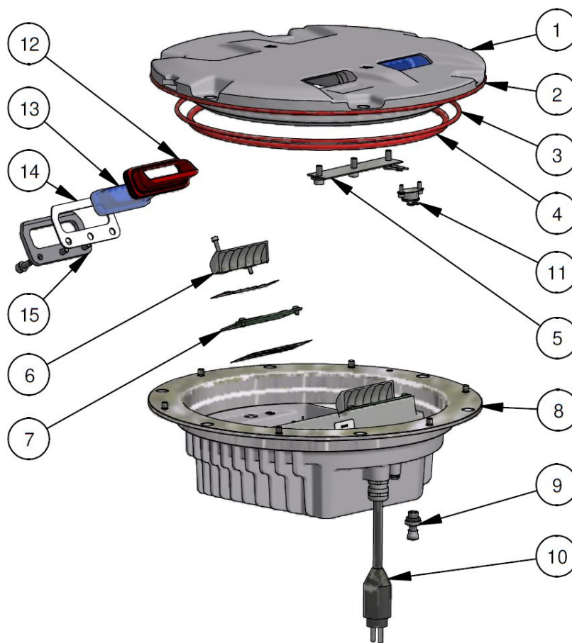
Figura 5 – Vista esplosa
