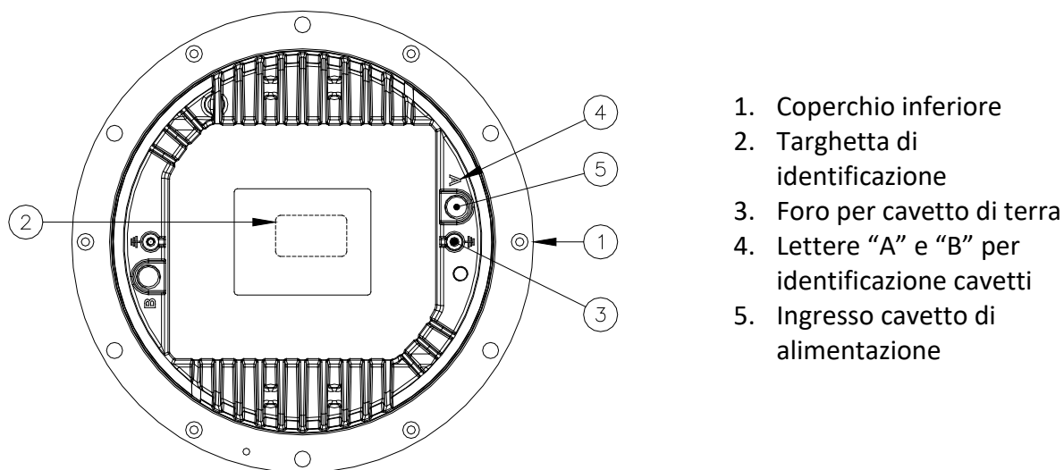
Figura 2 – Coperchio inferiore - vista esterna
