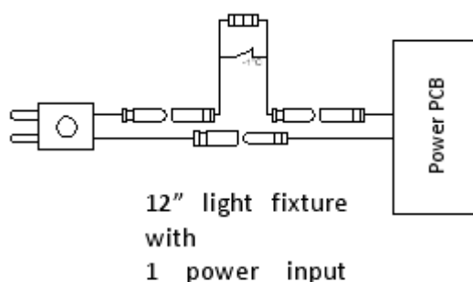
Figura 22 – Schema di collegamento elettrico del kit articolo
